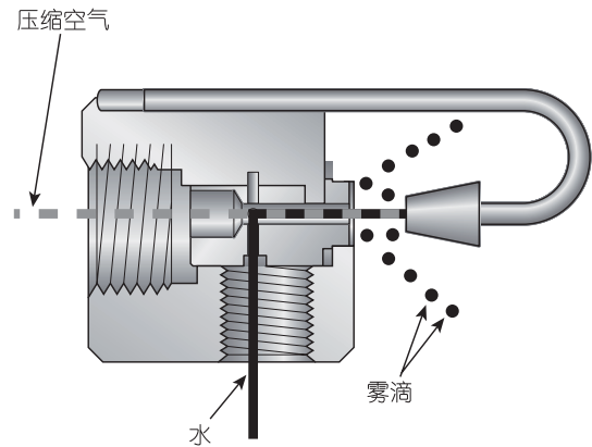
图151-2 加湿器喷雾头
